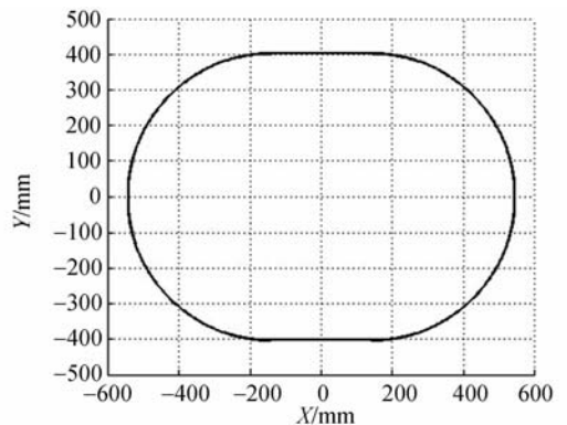
图 3 用于加工试验的 1 100 mm × 800 mm 体育场形工件的边界
