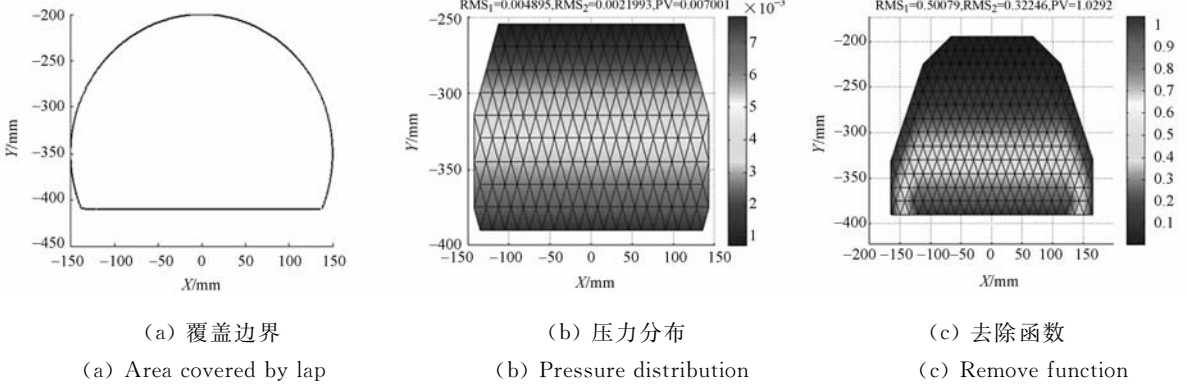
图 4 磨头处于图 3(0, -350)位置时的计算结果 Fig. 4 Calculation results when lap is at (0, -350) in Fig. 3
