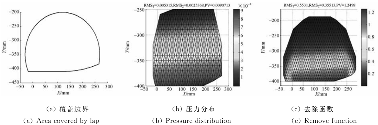
图 6 磨头处于图 3(125, -350)位置时的计算结果 Fig. 6 Calculation results when lap is at (125, -350) in Fig. 3
