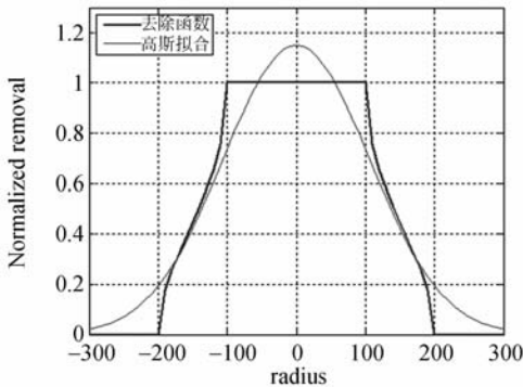
图 2 平转动方式的去除函数
