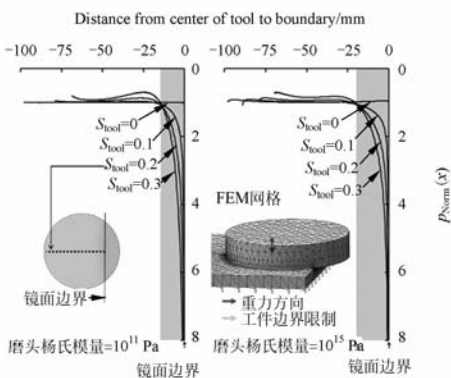
(b) 有限元模拟结果
